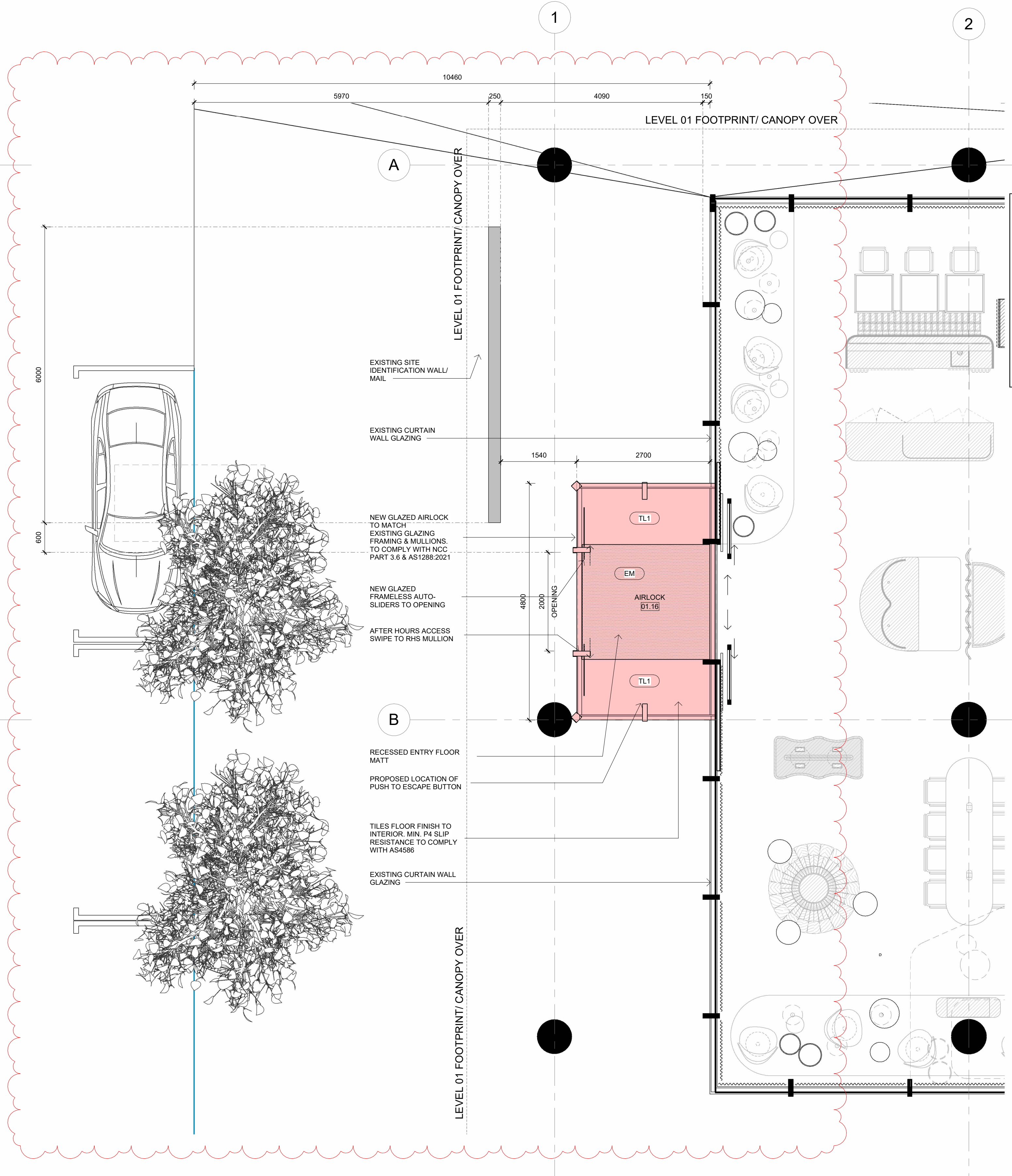
2 AIRLOCK DA GA PLAN 1:50
